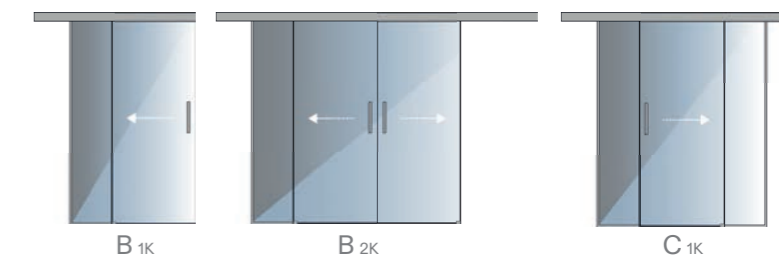
modelový rad SKLENENÉ POSUVNÉ STENY na stenu
